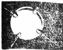
SPUTNIK 1 4 X 1957 415 kg prvi umjetni satelit
